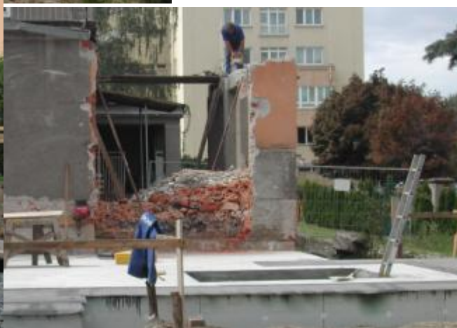
bourání verandy
